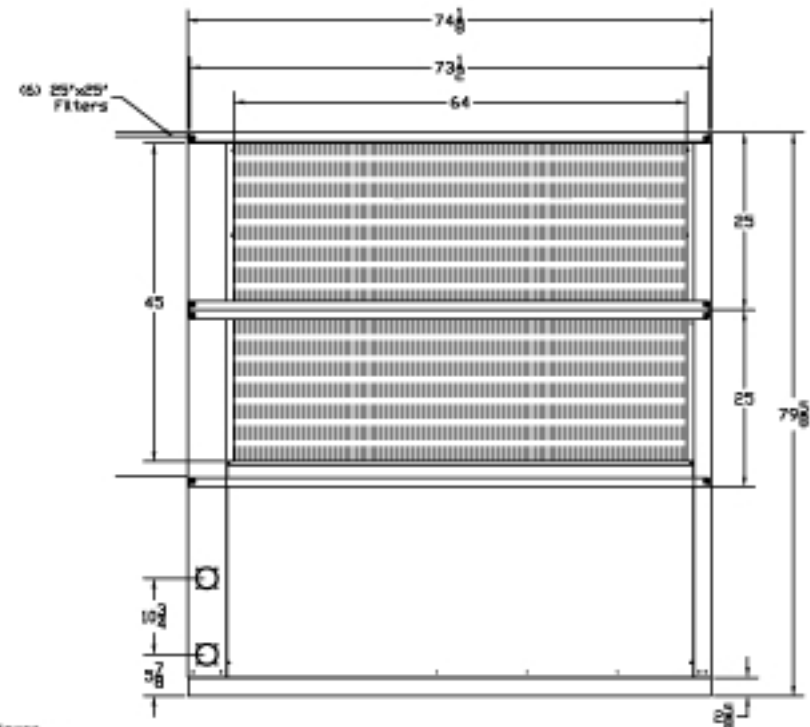
Elevation "C"
