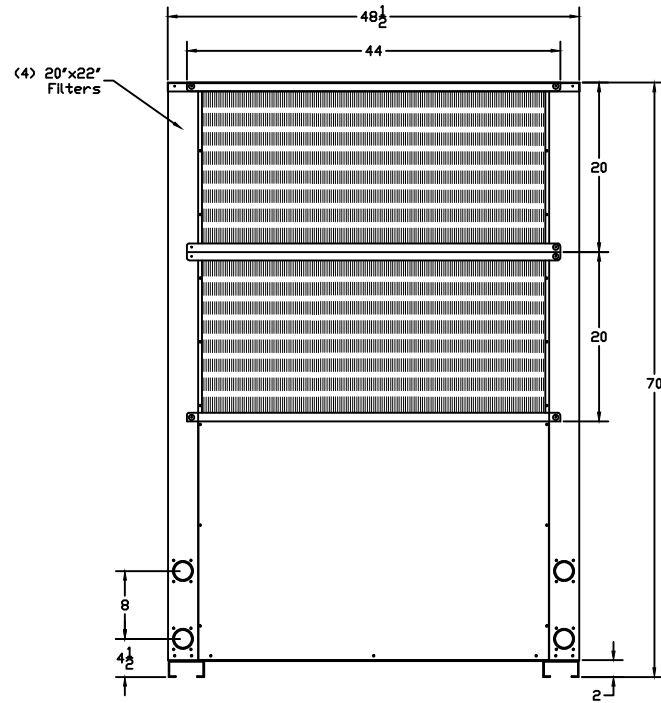
Elevation 'C'
