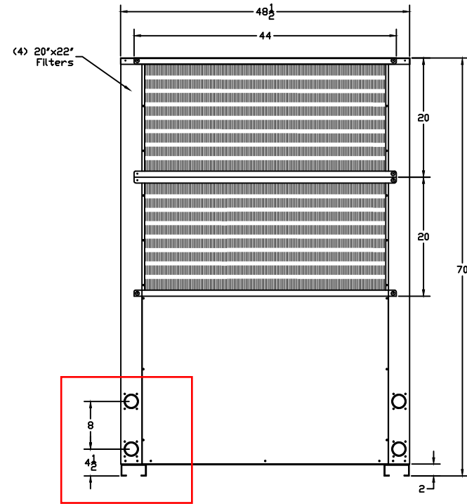
Elevation 'C'
